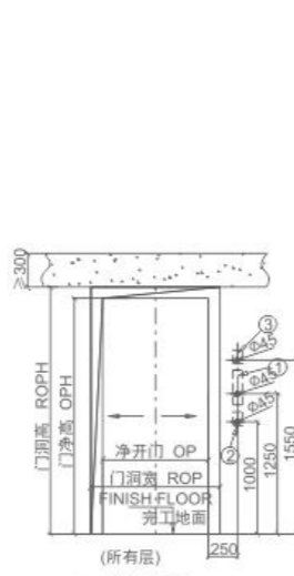
厅门图
