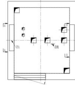
机房留孔图
