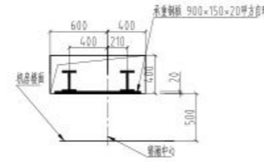
A-A承重孔
